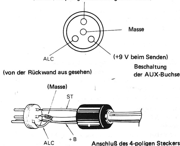
Fig. 3-8 Kontaktbelegung der AUX-Buchse
